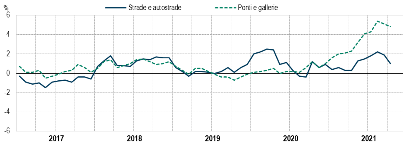
FIGURA 10. PREZZI ALLA PRODUZIONE DELLE COSTRUZIONI. STRADE E AUTOSTRADE, PONTI E GALLERIE Gennaio 2017 – ottobre 2021, variazioni percentuali tendenziali (base 2015=100)
